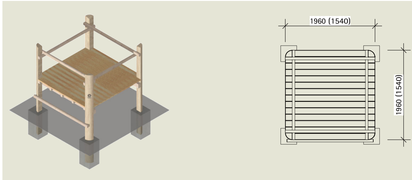
nuas® Plattform, groß/ klein
