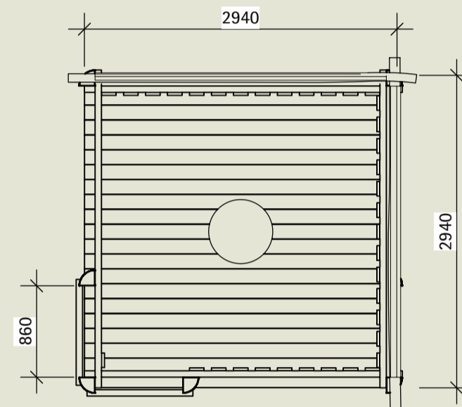
Plattform mit Rutsche, Balancierstamm und Brüstung
